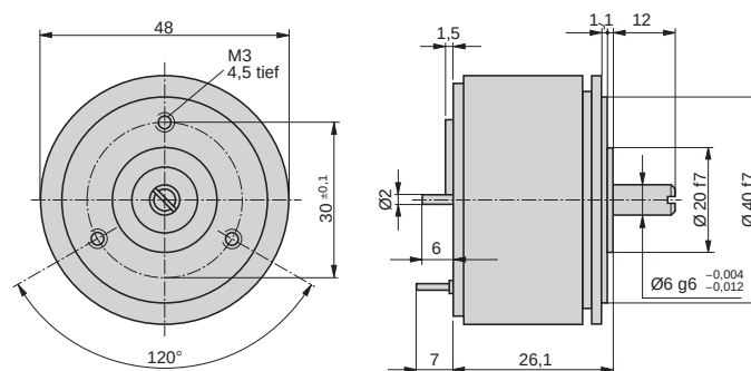
Bild 12. KINAX 2W2 mit Spezial-Antriebswelle vorn und hinten. Vorn: Ø 6 mm, Länge 12 mm. Hinten: Ø 2 mm, Länge 6 mm.
