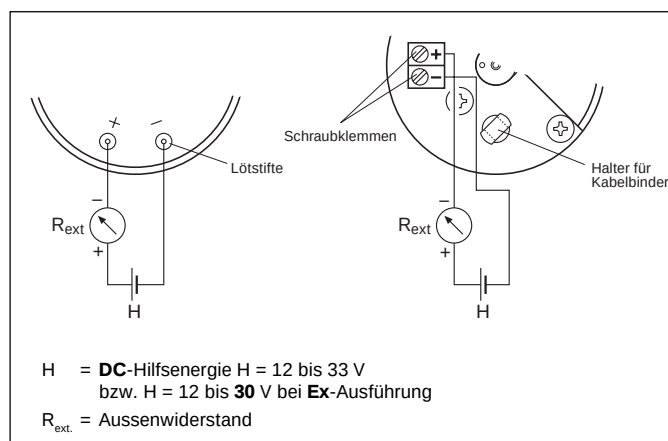
Bild 8. Anschlusspläne für 2-Drahtanschluss.
