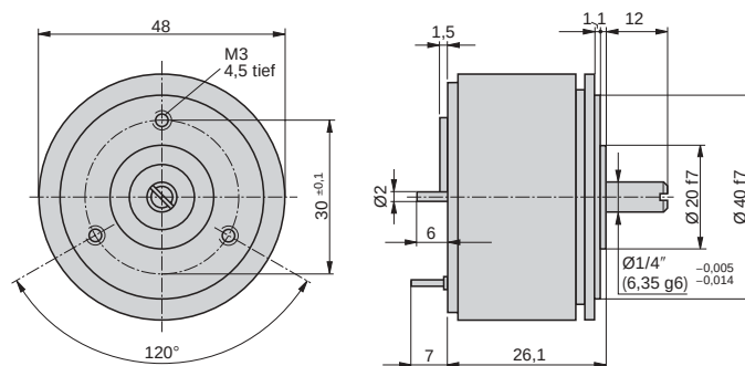
Bild 14. KINAX 2W2 mit Spezial-Antriebswelle vorn und hinten. Vorn: Ø 1/4", Länge 12 mm. Hinten: Ø 2 mm, Länge 6 mm.
