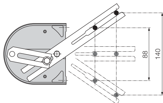
Bild 4. Maximale Hubeinstellung am Anschlusshebel.
