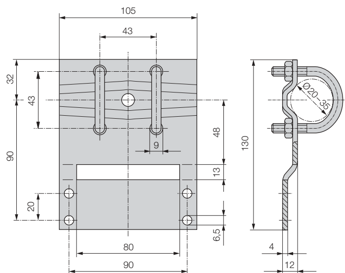
Bild 12. NAMUR-Anbausatz.
