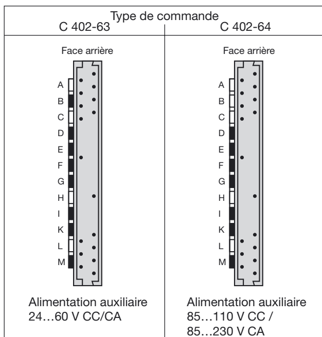
Fig. 5. Codage du module embrochable SIRAX C 402 en exécution [Ex ia] IIC.
