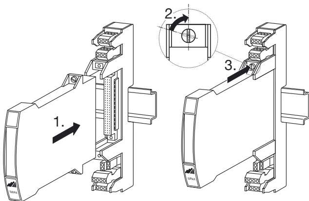
Bild 7. Steck-Modul aufstecken.
