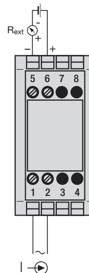
Bild 4. Speisung über Ausgangskreis.
