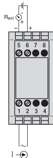
Fig. 4. Alimentation à travers le circuit de sortie.
