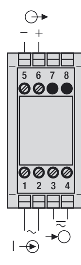
Fig. 5. Alimentation auxiliaire CC, CA en exécution avec bloc d'alim. CC, CA incorporé.
