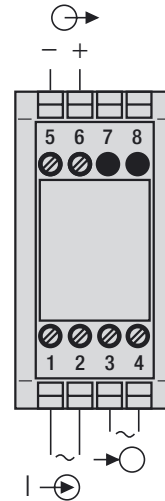
Bild 2. AC-Hilfsenergie.
