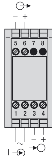
Fig. 3. Alim. auxiliaire CC.
