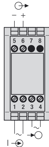
Fig. 2. Alim. auxiliaire CA.
