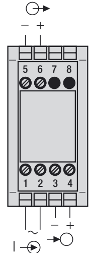
Bild 3. DC-Hilfsenergie.
